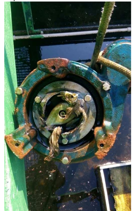
Kalové čerpadlo s řezacím nožem zanesené hadry a igelitem
